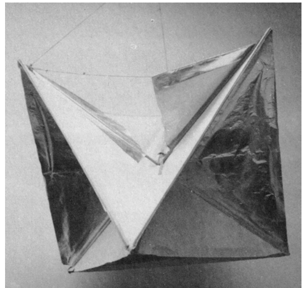
Radar-Reflektor vom Typ ML-307 AP, von dem es die Varianten A, B, C u. D gab
