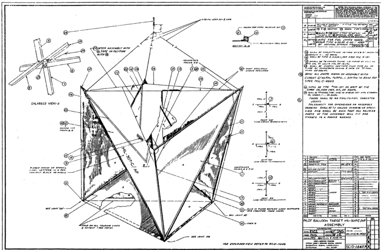
Skizze eines beim Projekt MOGUL benutzten Radarreflektor vom Typ ML-307
