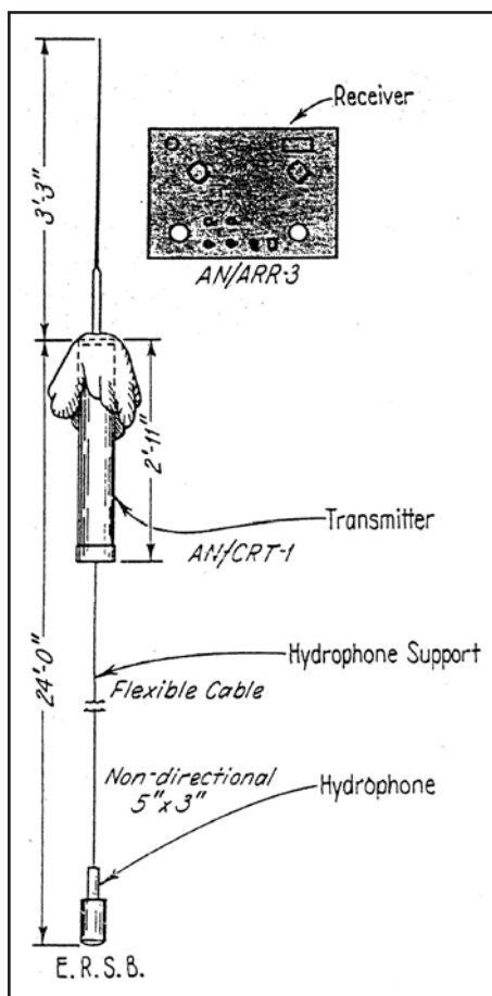
Skizze einer AN/CRT-1 Sonarboje die eine Länge von 2 Foot 11 Inch [87 cm] hatte.
