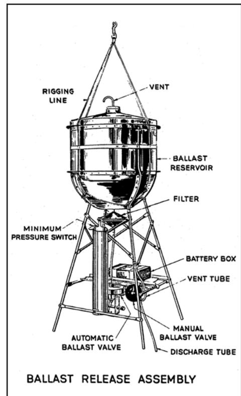
Ballast-Abwurf-Konstruktion mit der "Black Box", der Batterie Schachtel
